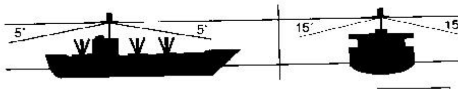
Disposition d'antenne INMARSAT C 1
